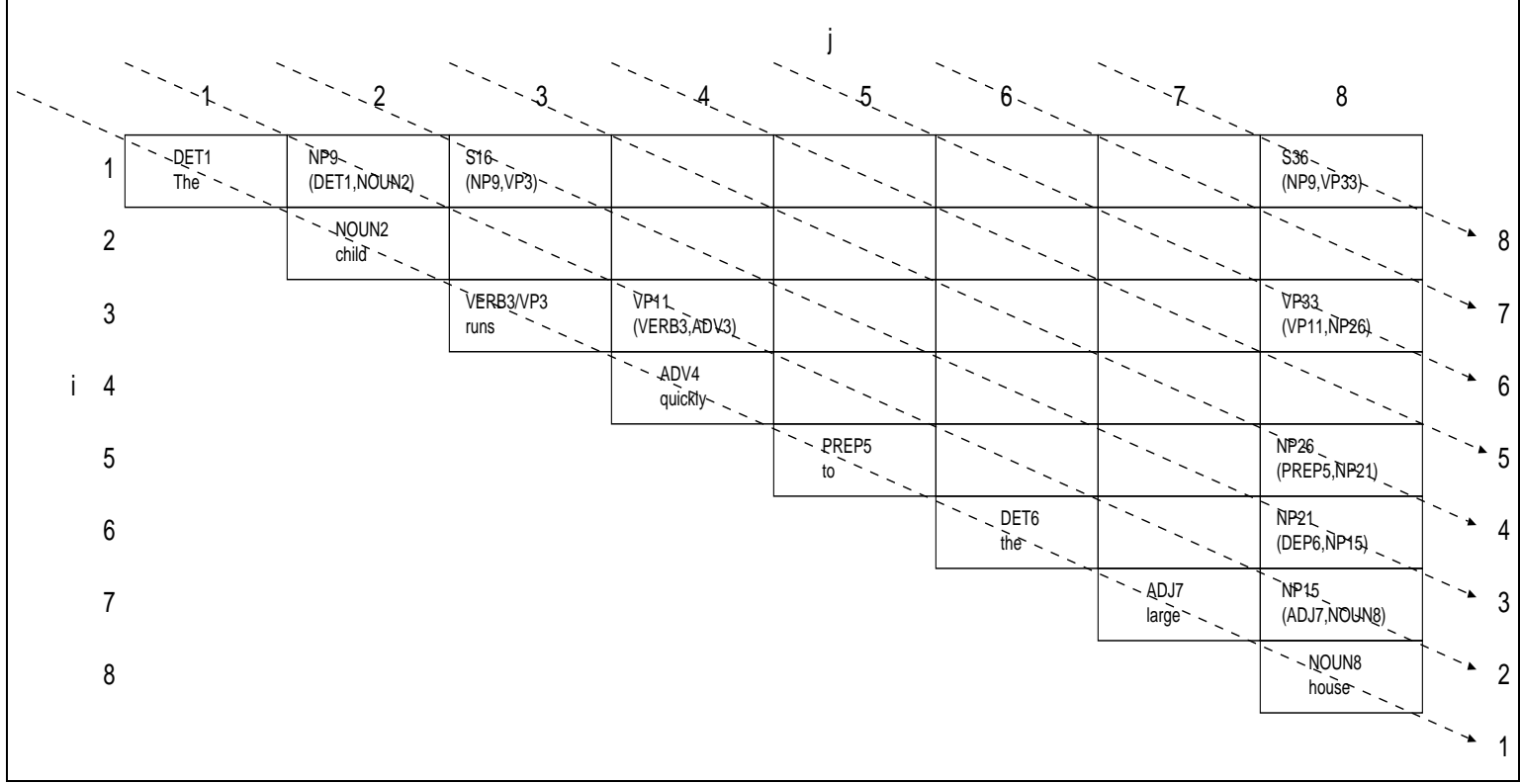
図 5. CKY パーザの動作
