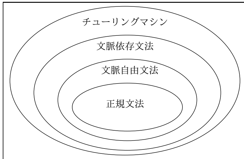
図 1: チョムスキーの言語階層
